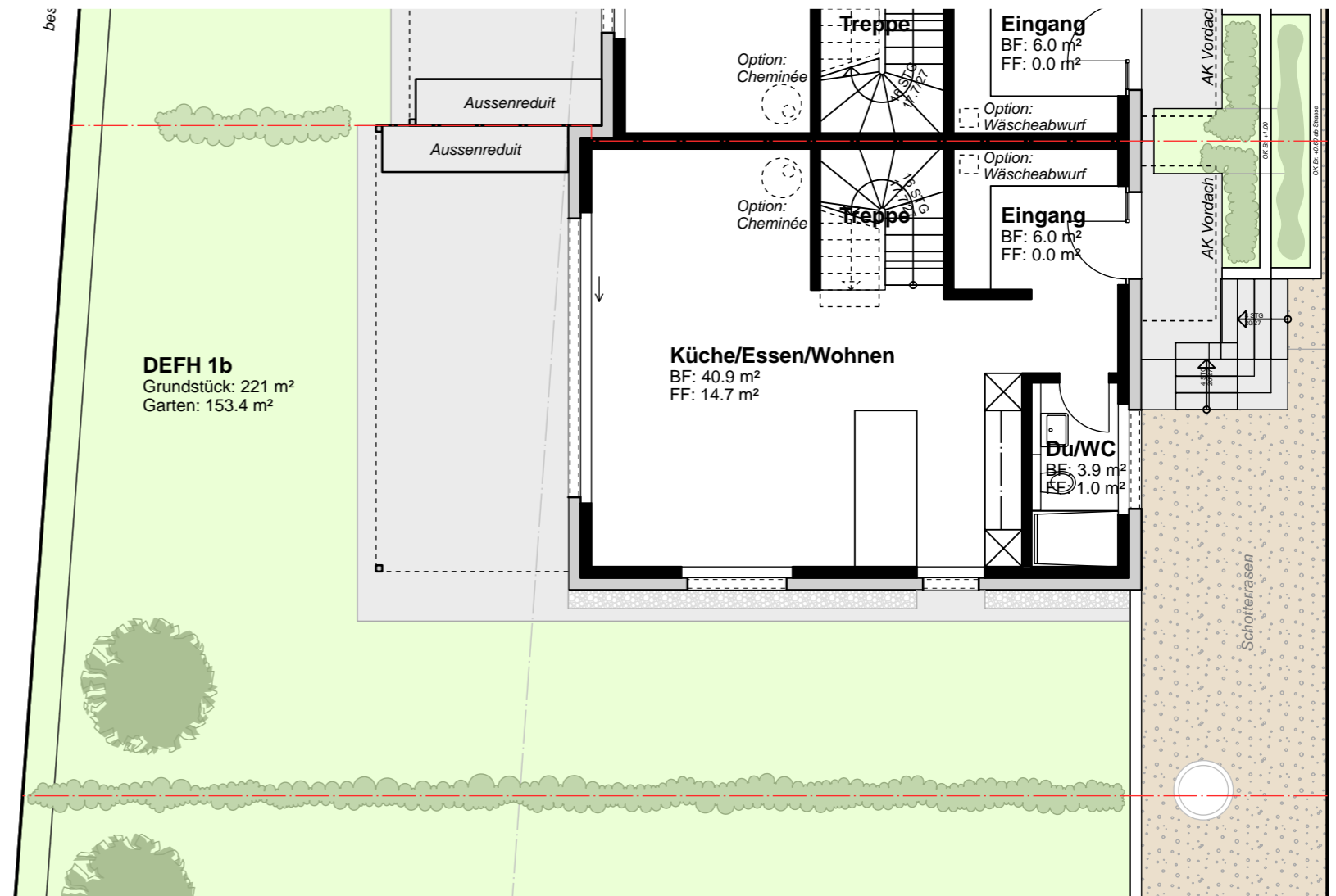
Grundriss Erdgeschoss
