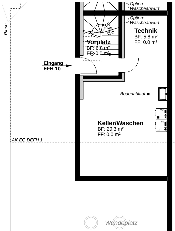
Grundriss Kellergeschoss
