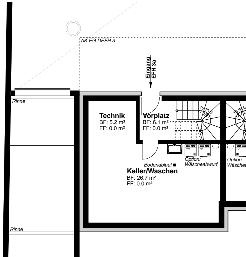
Grundriss Kellergeschoss
